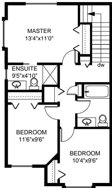
UPPER FLOOR 668 SQ.FT
